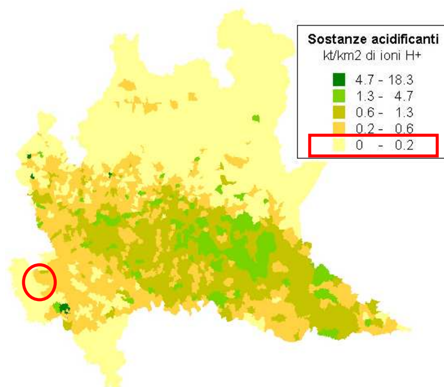
Figura 68: Acidificanti (2010)
